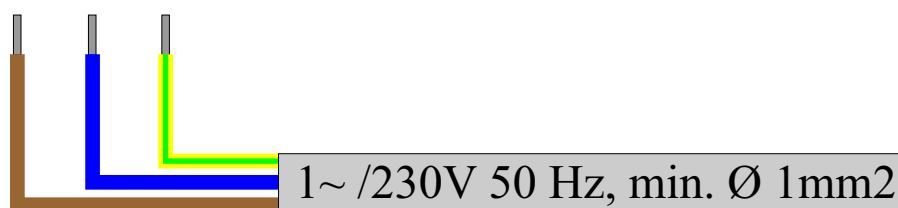
Podłączenie siłownika TECHNIX
