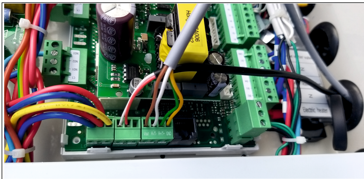
Miejsce podłączenia wtyczki z przewodem z panelu sterującego w pompie ciepła
